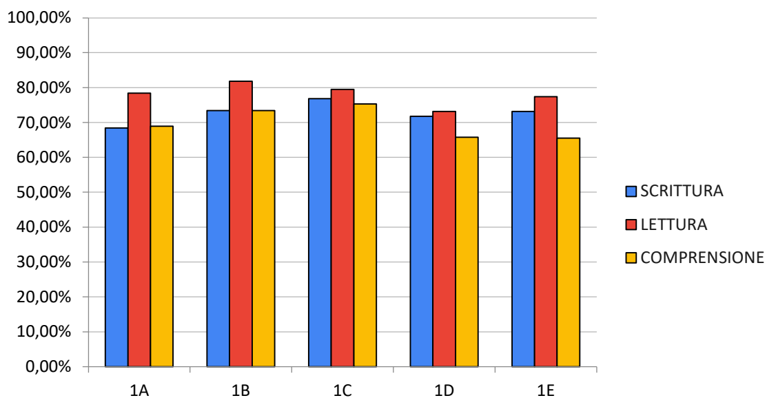
Prova di Uscita Italiano - Confronto fra le classi
