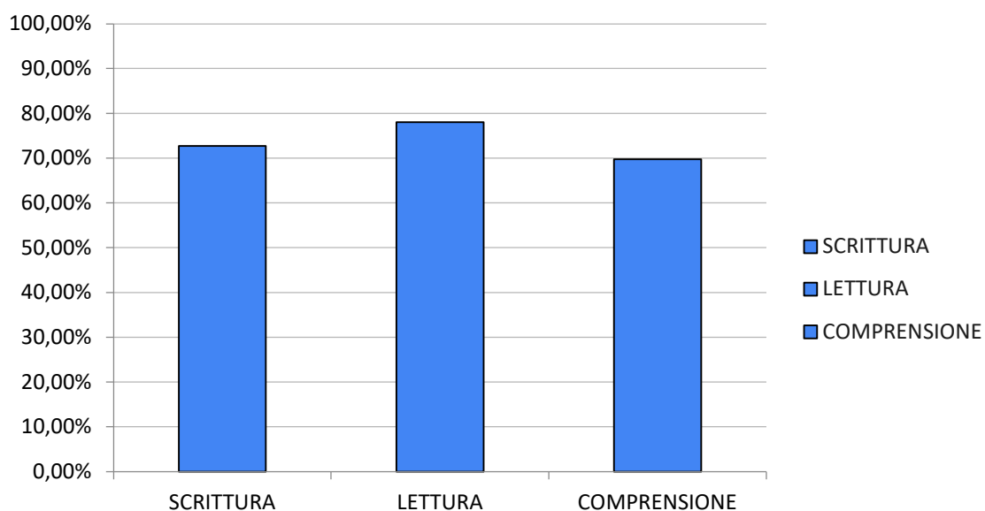
Andamento medio italiano classi prime
